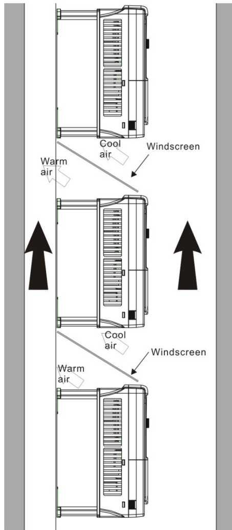
Рис. 4-5 Вертикальная установка
