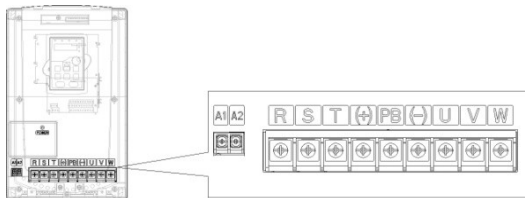
Рис. 4-11. 18,5 кВт клеммы силовых цепей
