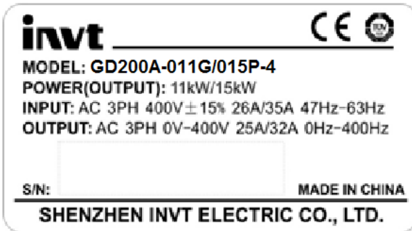
Рис. 3-3 Табличка ПЧ
