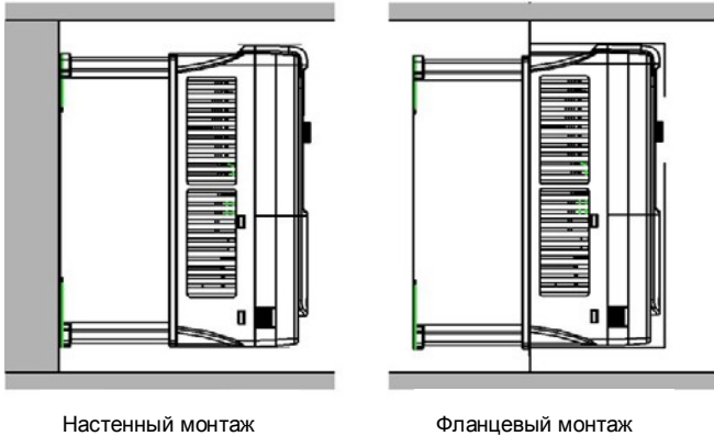
Рис. 4-2 Способ установки
