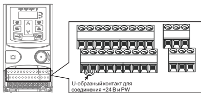
Рис.5-18 U-образный контакт
