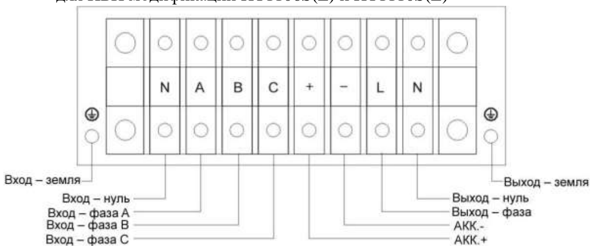
Рисунок 3.2 - Схема соединения блока входных и выходных клемм для ИБП модификаций NT3110L, NT3112L, NT3115L или NT3120L
