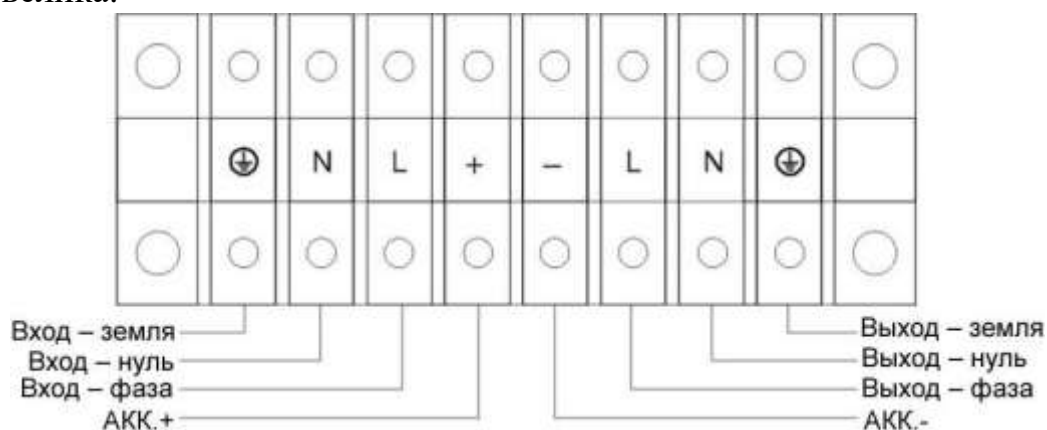
Рисунок 3.1 - Схема соединения блока входных и выходных клемм для ИБП модификаций NT1106S(L) и NT1110S(L)
