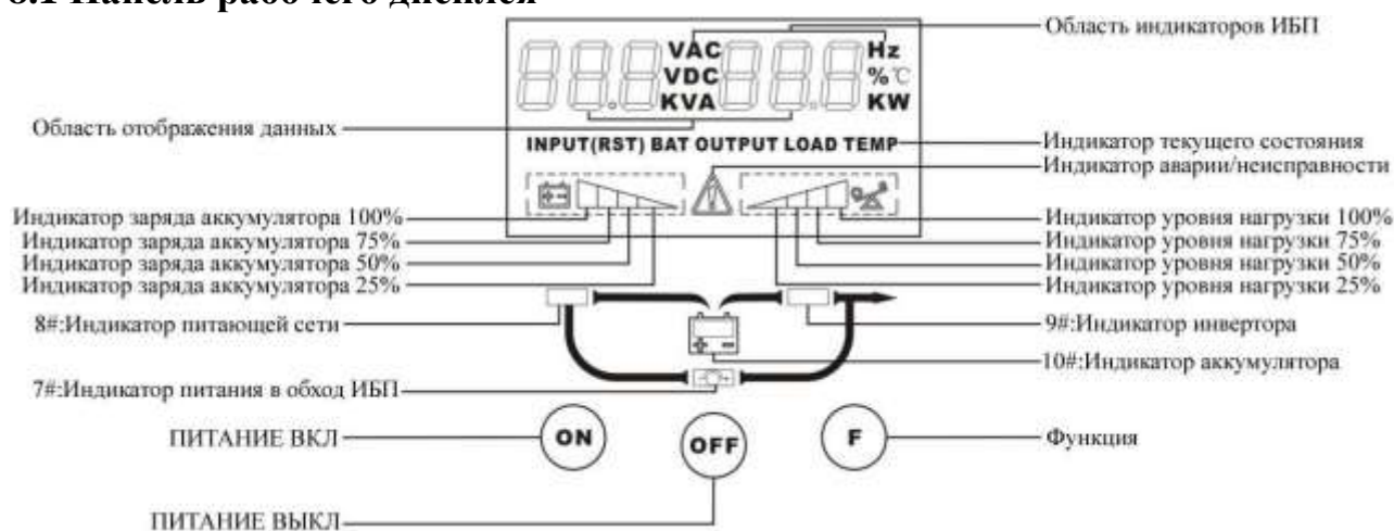
Рисунок 8.1 – ЖК-дисплей
