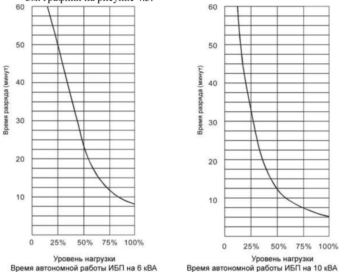
Рисунок 4.5 - Время автономной работы для стандартных ИБП
